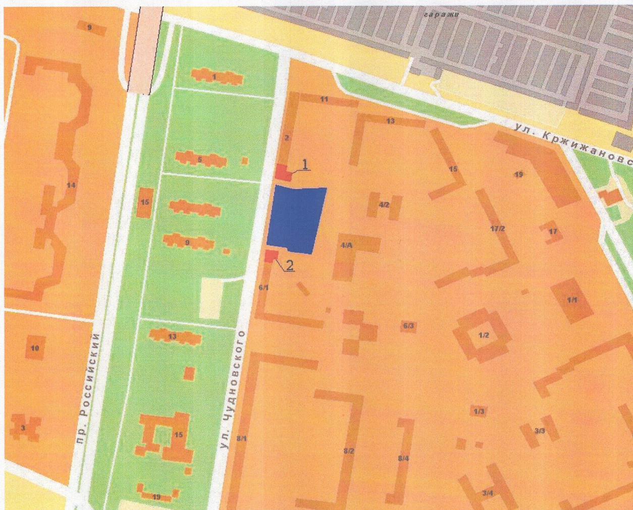
Рис. 2.1. Ситуационный план (граница участка предполагаемого строительства центра социальной реабилитации инвалидов и детей-инвалидов выделена синим цветом, обследуемые секции зданий окружающей застройки – красным цветом): 1. Южная торцевая секция жилого дома по адресу: ул. Чудновского, дом 2; 2. Северная торцевая секция жилого дома по адресу: ул. Чудновского, дом 6, корпус 1.
